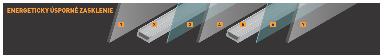
1: 3 mm tvrdené bezpečnostné sklo 2, 5: Komora plnená argónom 3, 6: Nízkoemisná povrchová vrstva [odráža teplo] 4: 3 mm kalené sklo 7: 4 mm číre sklo
