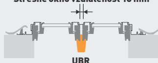
Strešné okno vzdialenosť 18 mm
